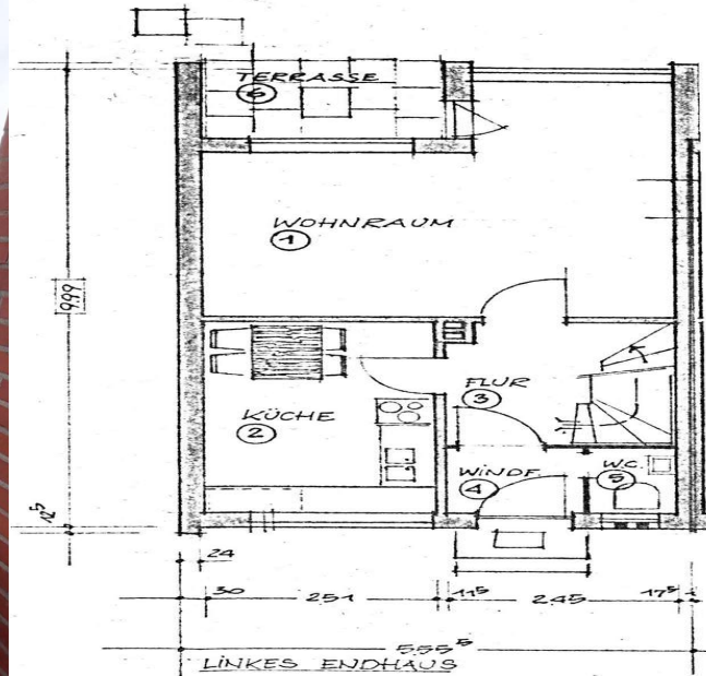
ERDGESCHOSS - GRUNDRISS
