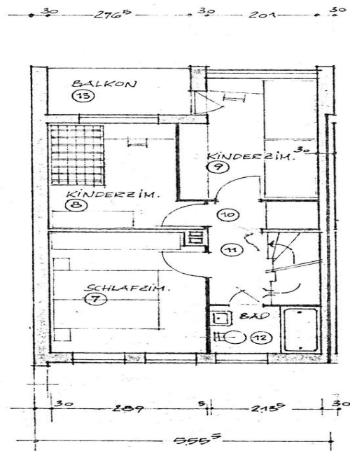
OBERGESCHOSS - GRUNDRISS
