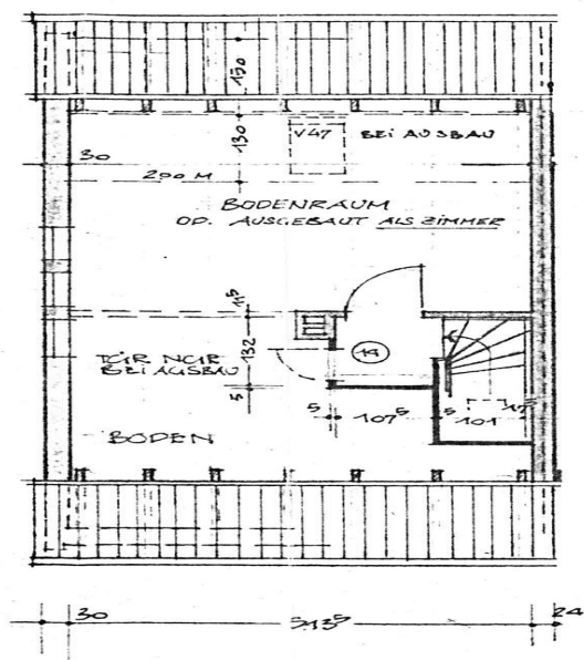
LINKES ENDHAUS
