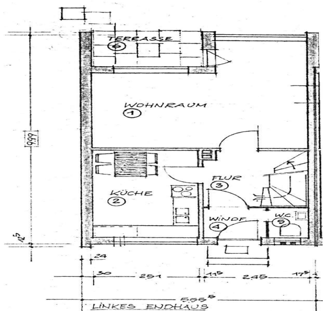
ERDGESCHOSS - GRUNDRISS
