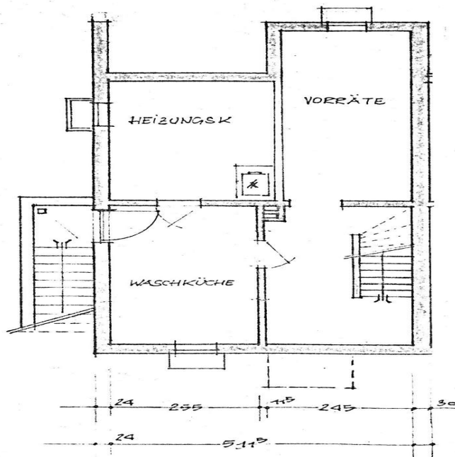
KELLERGRUNDRISS
